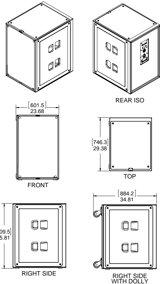
S2-A Sub EP-8 Pin Configuration
